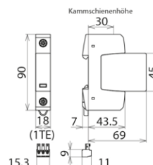
Maßbild DSIT S CSP DC 48 FM
