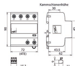
Maßbild DVA CSP 3P 100 S FM
