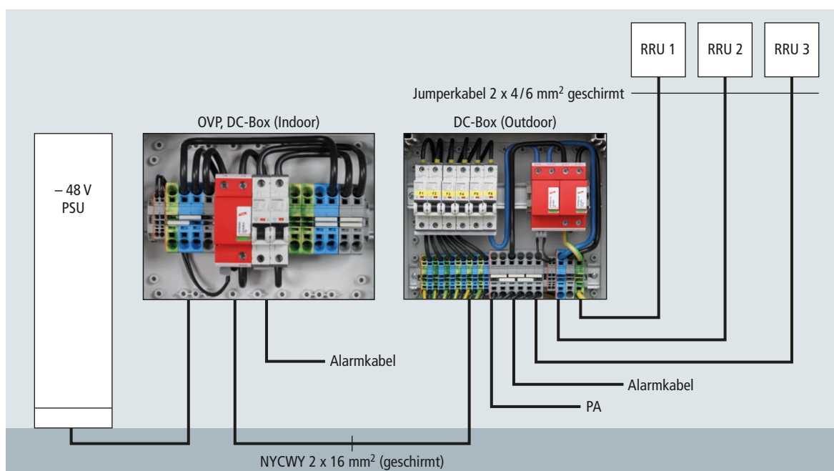
Bild 6 Schaltbild von Remote Radio Heads (RRHs) bei räumlich getrennten Funktionspotentialausgleichsebenen mit DC-Box (Outdoor) und DEHNsecure DSE M 2P 60 FM sowie OVP-Box (Indoor) und DEHNsecure DSE M 1 60 FM
