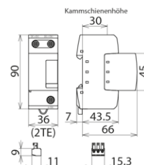
Maßbild DSE M 1 60 FM
