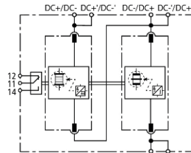
Prinzipschaltbild DSE M 2P 60 FM
