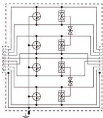
Prinzipschaltbild DPA CLE IP66
