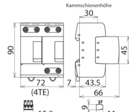
Maßbild DSE M 2P 60 FM
